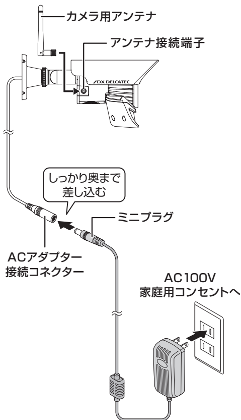
カメラ用ACアダプター
